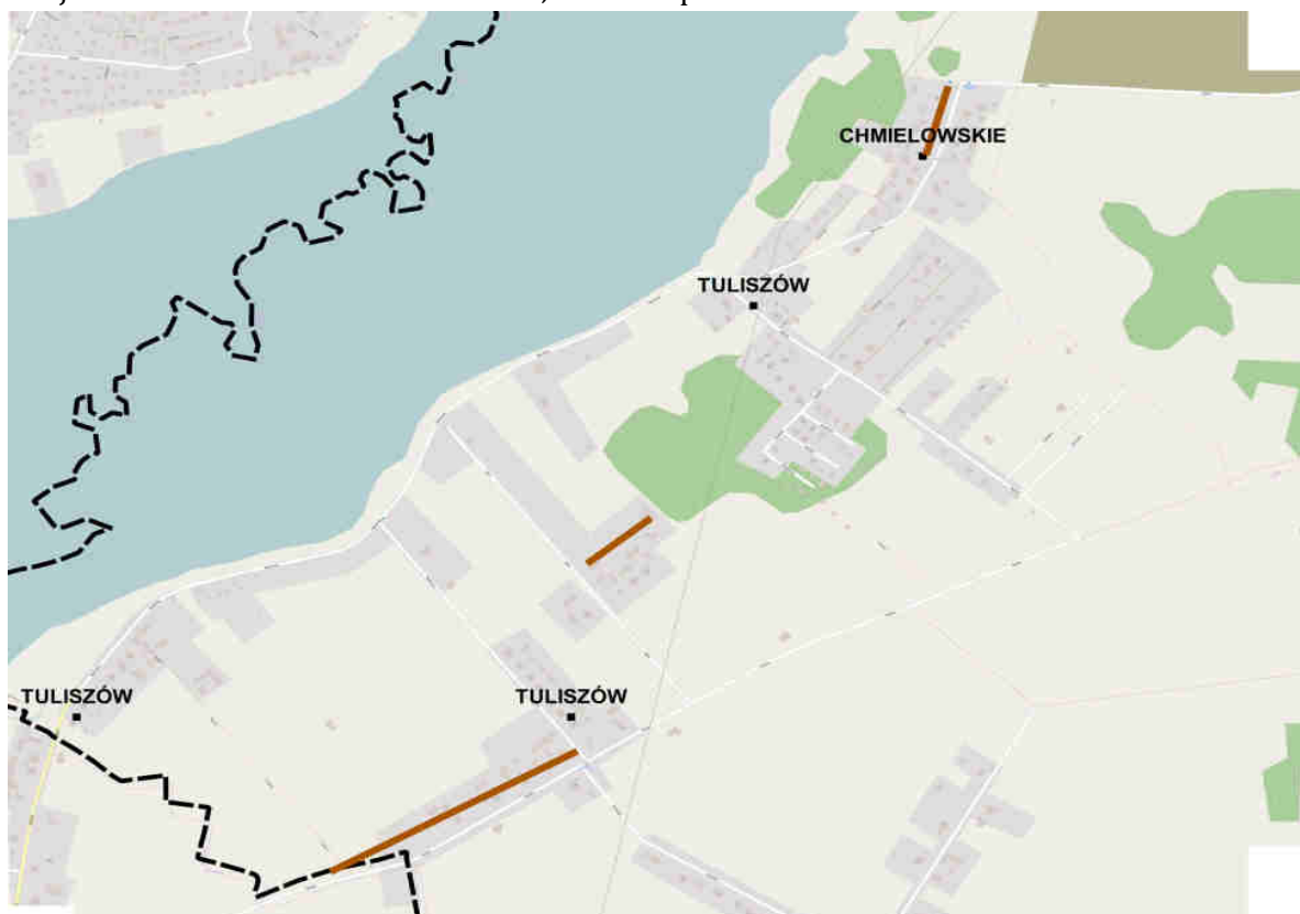
Rysunek 7. Lokalizacja rur azbestowo-cementowych sieci wodociągowej (linia brązowa) w obrębie miejscowości Tuliszków i Chmielowskie, stan na lipiec 2015r.
