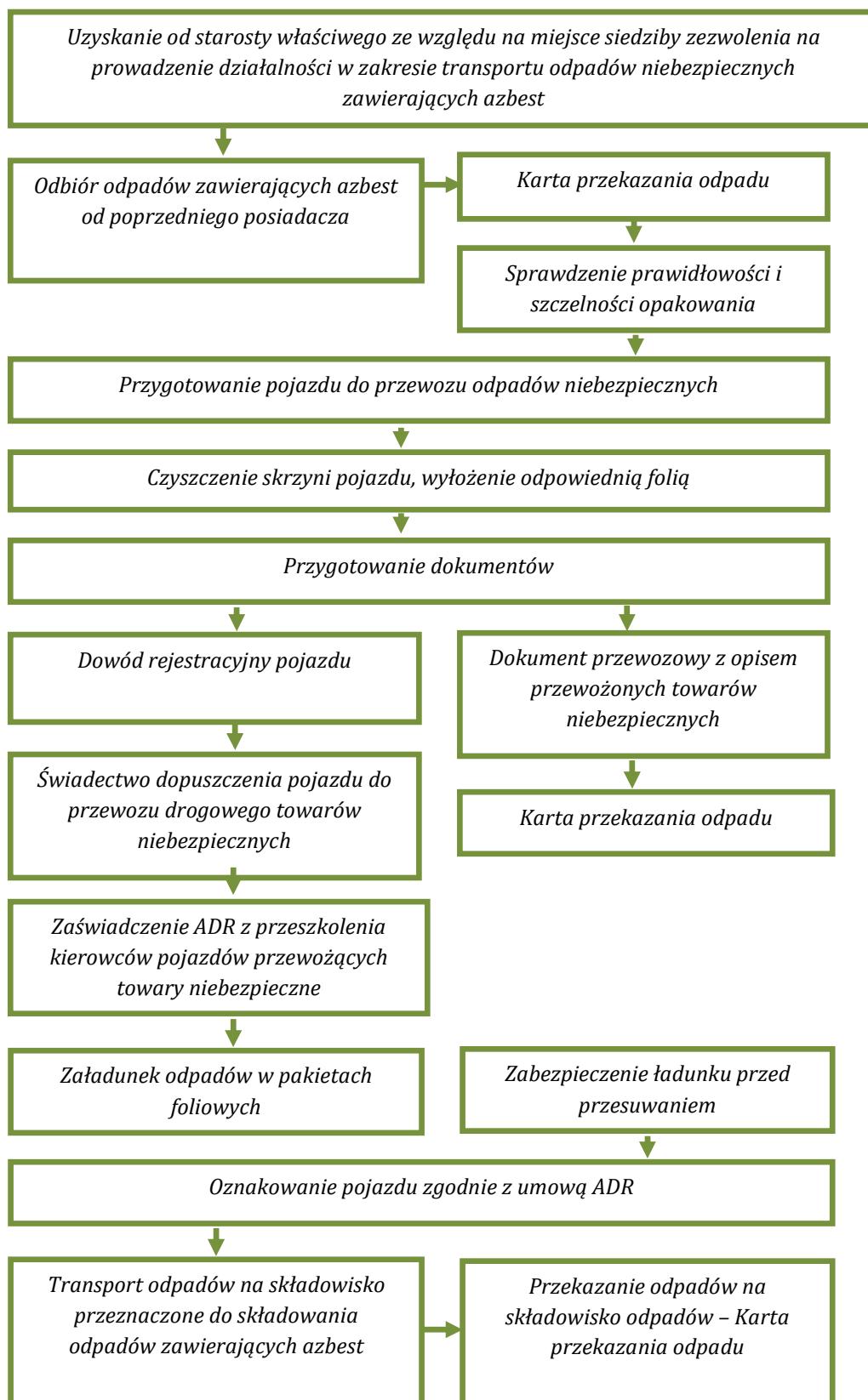
Rysunek 11. Procedura 5 - Przygotowanie i transport odpadów niebezpiecznych zawierających azbest
