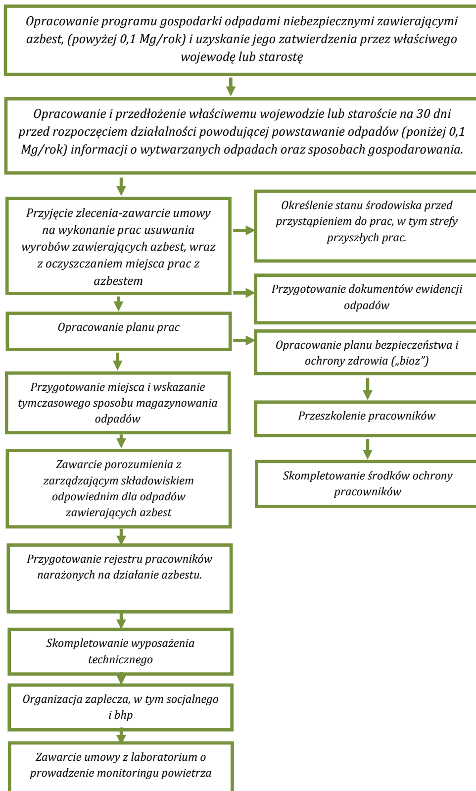
Rysunek 10. Procedura 3 - Postępowanie przy pracach przygotowawczych do usuwania wyrobów zawierających azbest.
